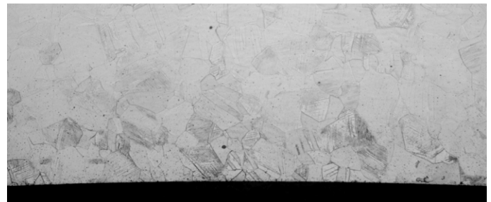
Figura 6. Expansión con Pasador Cónico con una Reducción del 6 % del Espesor de Pared
