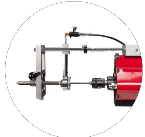
Cómo Expansionar Cada Tubo De Manera Consistente
